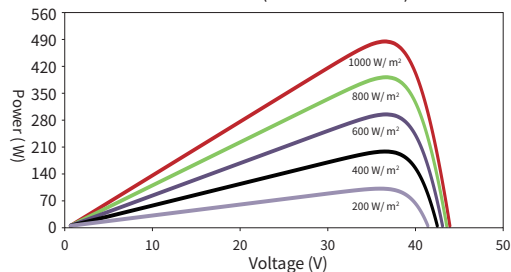
出力-電圧曲線 (54HL4R-B 430W)
