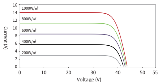
電流-電圧曲線 (54HL4R-B 430W)
