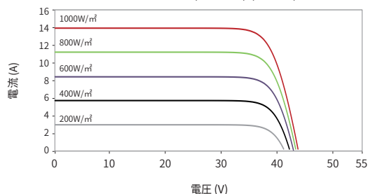
電流-電圧曲線 (60HL4-(V) 480W)
