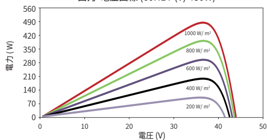
出力-電圧曲線 (60HL4-(V) 480W)
